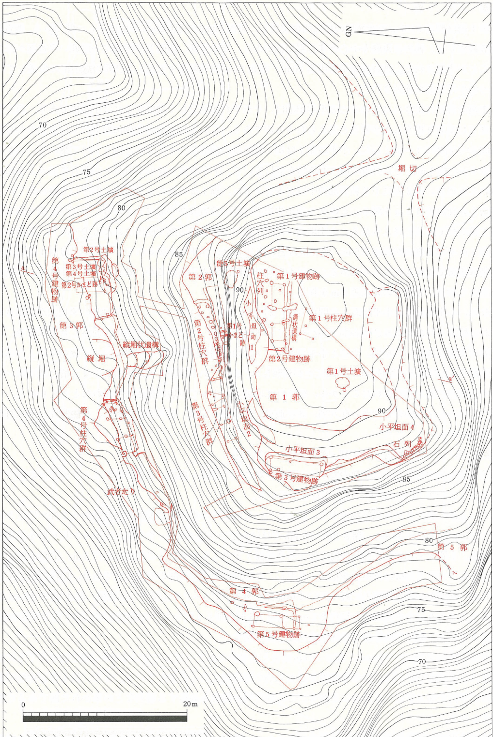
北谷山城跡地形測量図及び遺構配置図
