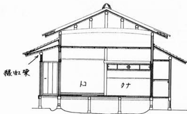
後方角家 座敷断面図
