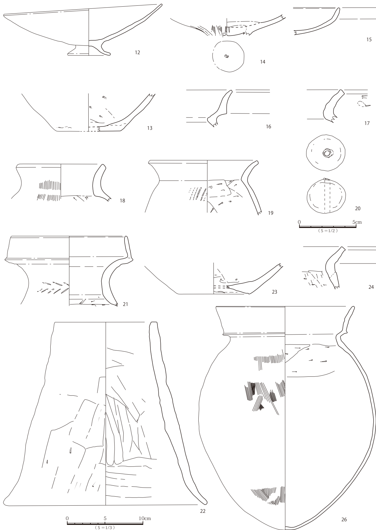
第 61 図 出土遺物実測図 (2) (S=1/3, 20 は S=1/3)
