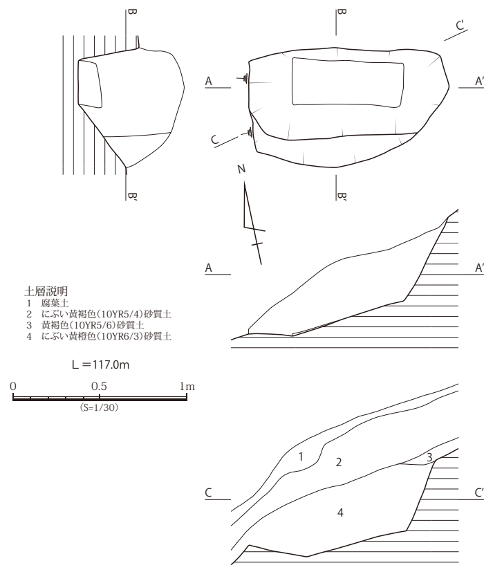
第 109 図 坊主山遺跡 ST21 実測図 (S=1/30)
