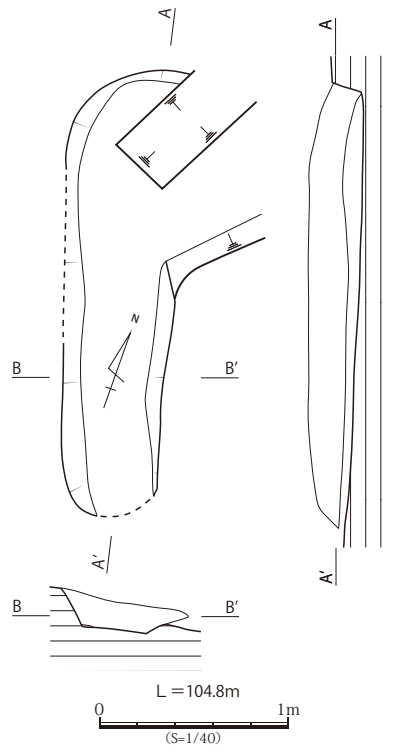
第 54 図 ST9 実測図 (S=1/40)
