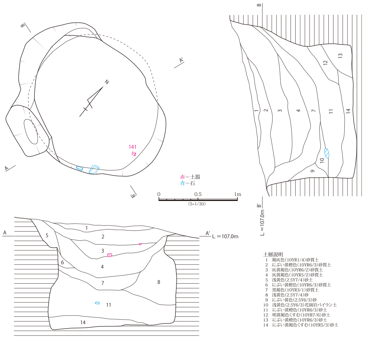
第 40 図 トンガ坊城遺跡 SK12 実測図 (S=1/30)
