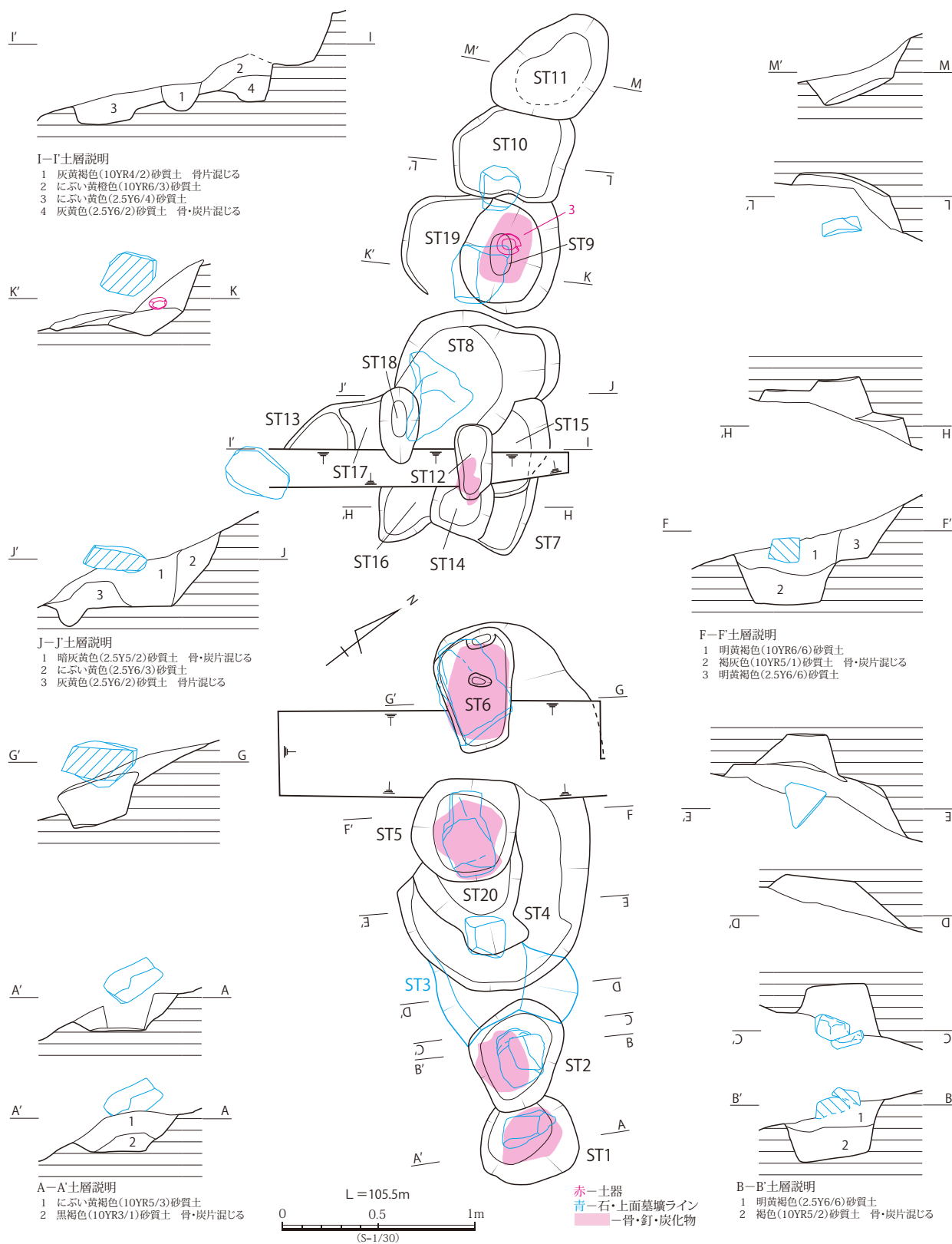
第 87 図 火葬墓群 (ST1 - 20) 実測図 (S=1/30)
