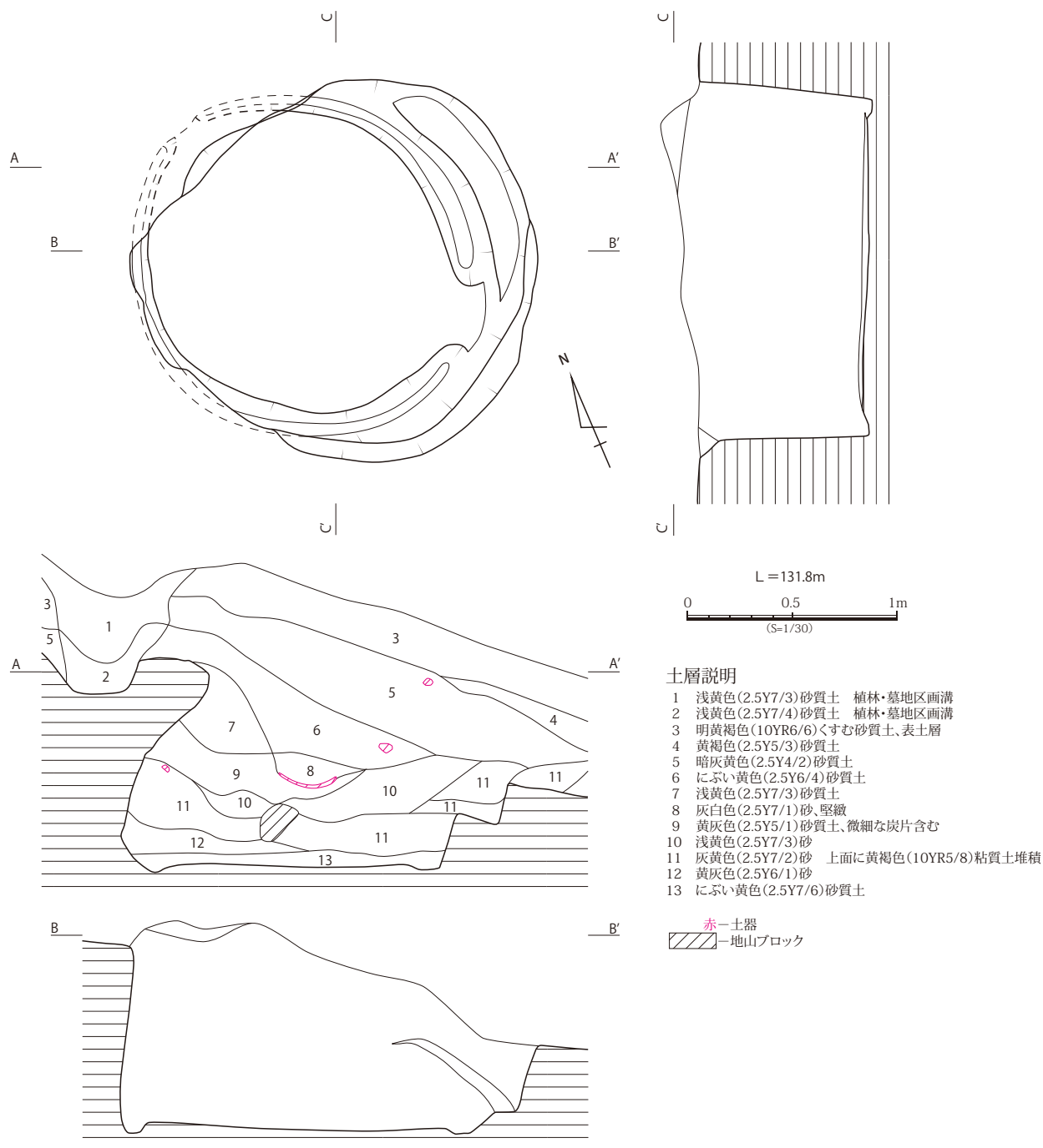
第 142 図 柳遺跡 SK3 実測図 (S=1/30)
