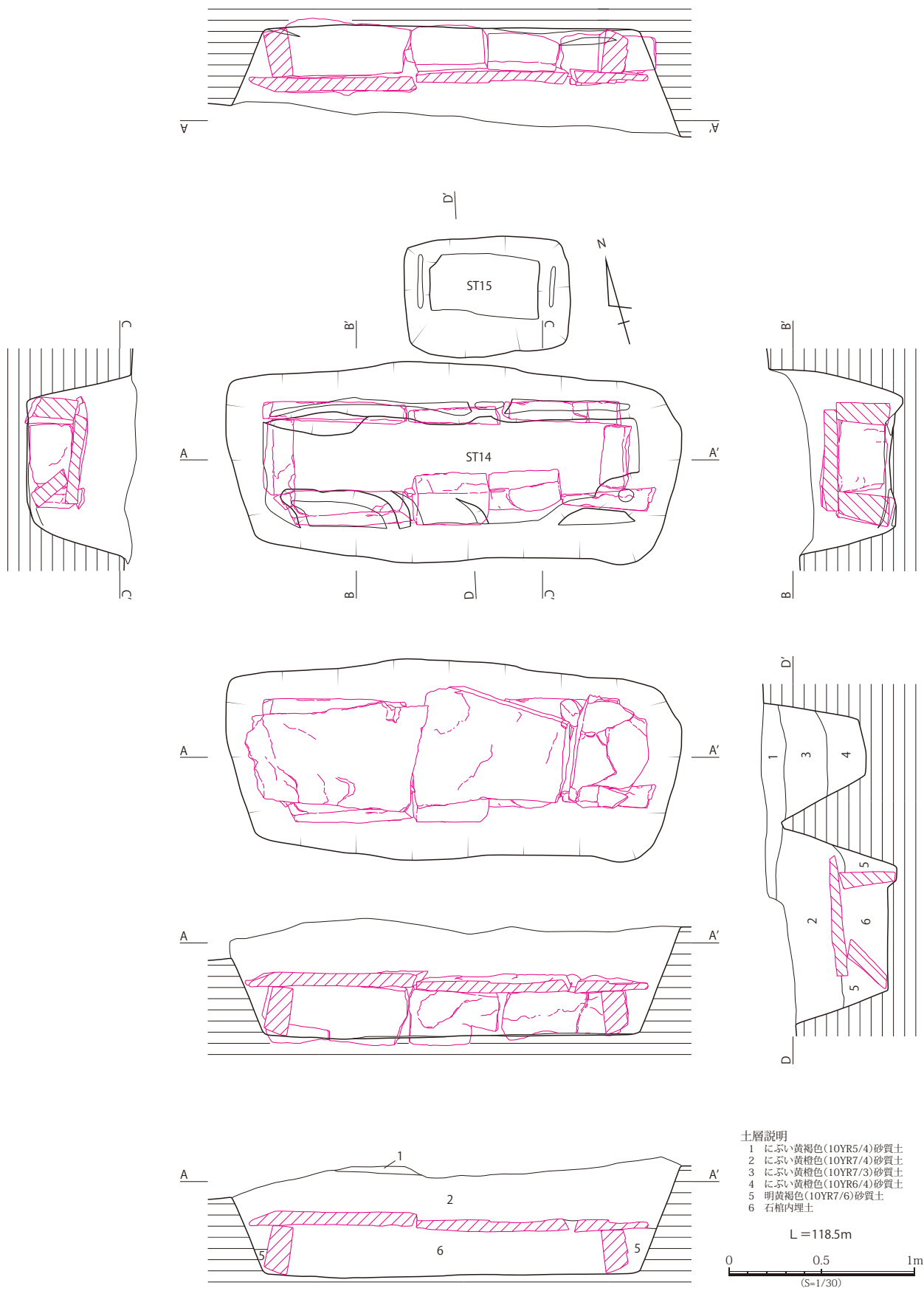
第 103 図 坊主山遺跡 ST14 実測図 (S=1/30)
