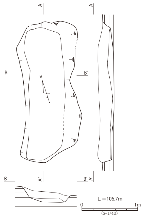
第51図 ST6 実測図 (S=1/40) 第52図 ST7 実測図 (S=1/40) 第53図 ST8 実測図 (S=1/40)
