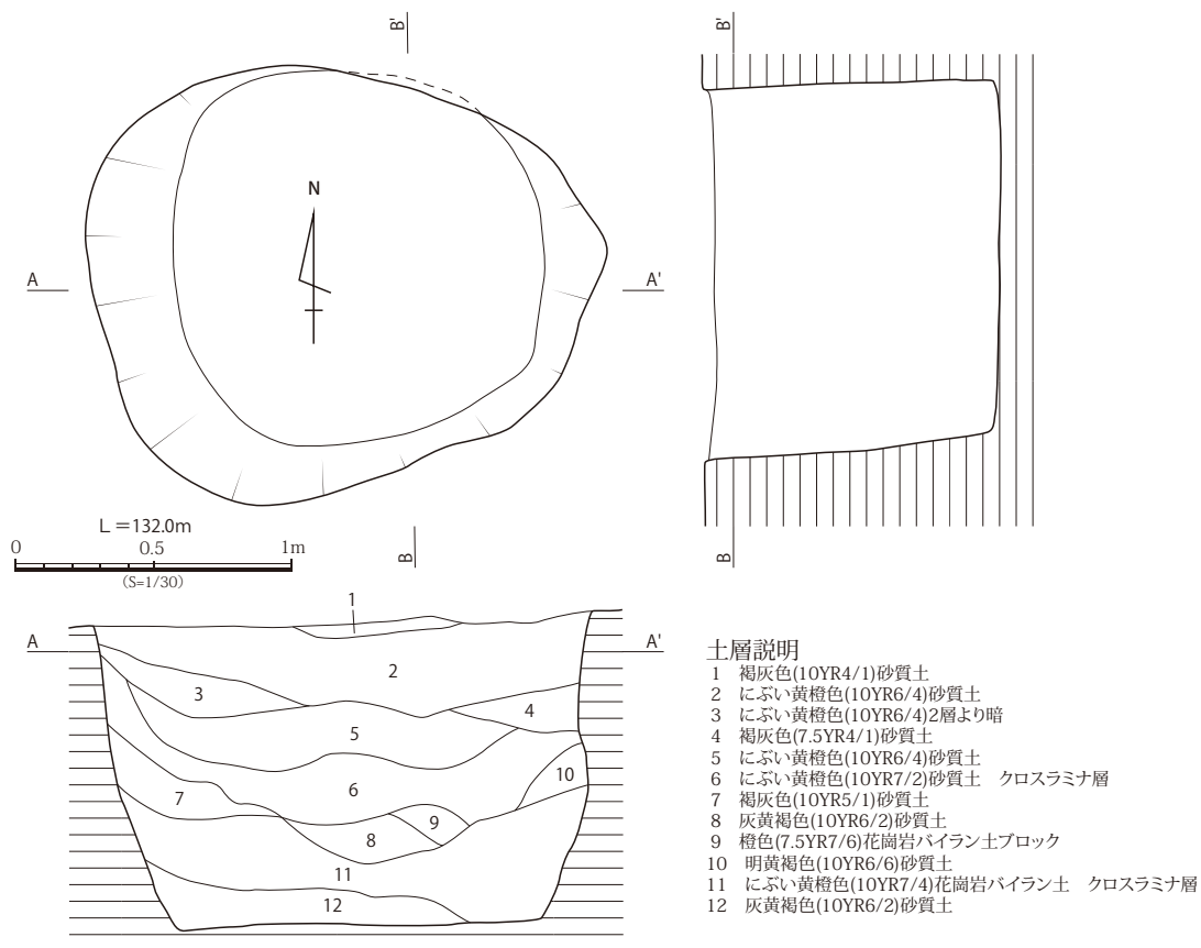
第 140 図 柳遺跡 SK1 実測図 (S=1/30)
