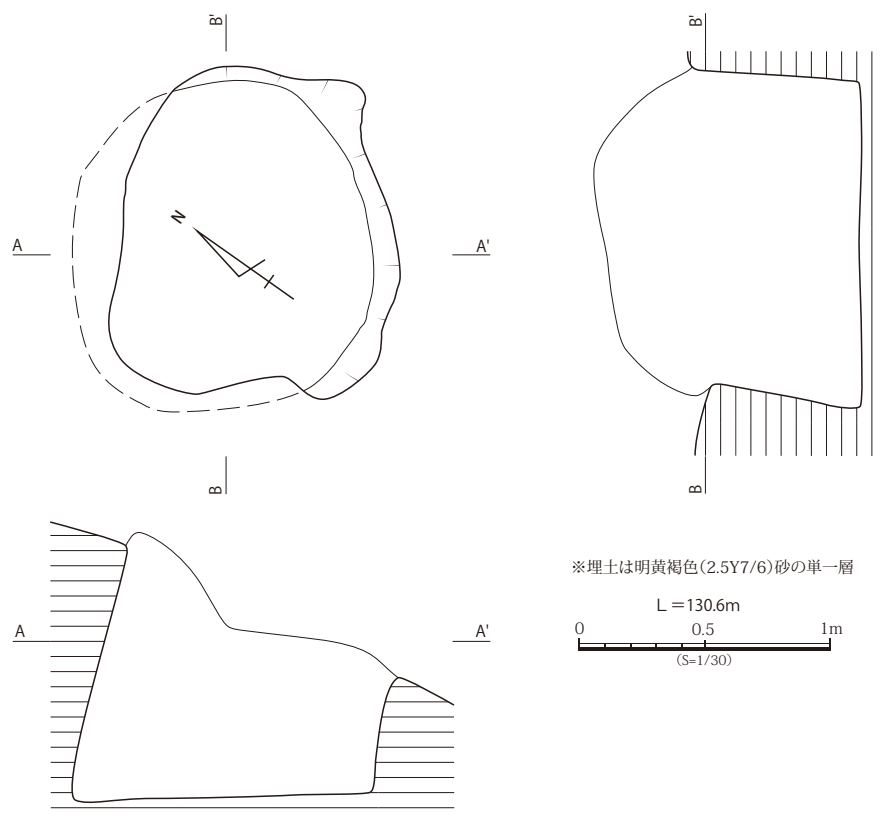
第 145 図 柳遺跡 SK7 実測図 (S=1/30)
