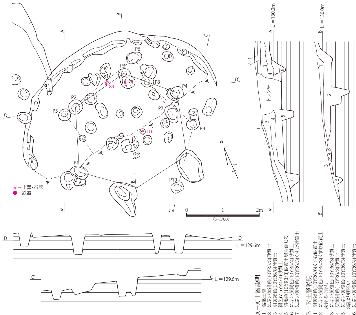
第 128 図 柳遺跡 SH4 実測図 (S=1/60)
