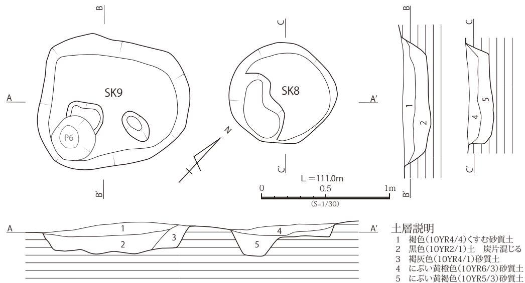
第 31 図 トンガ坊城遺跡 SK8・SK9 実測図 (S=1/30)
