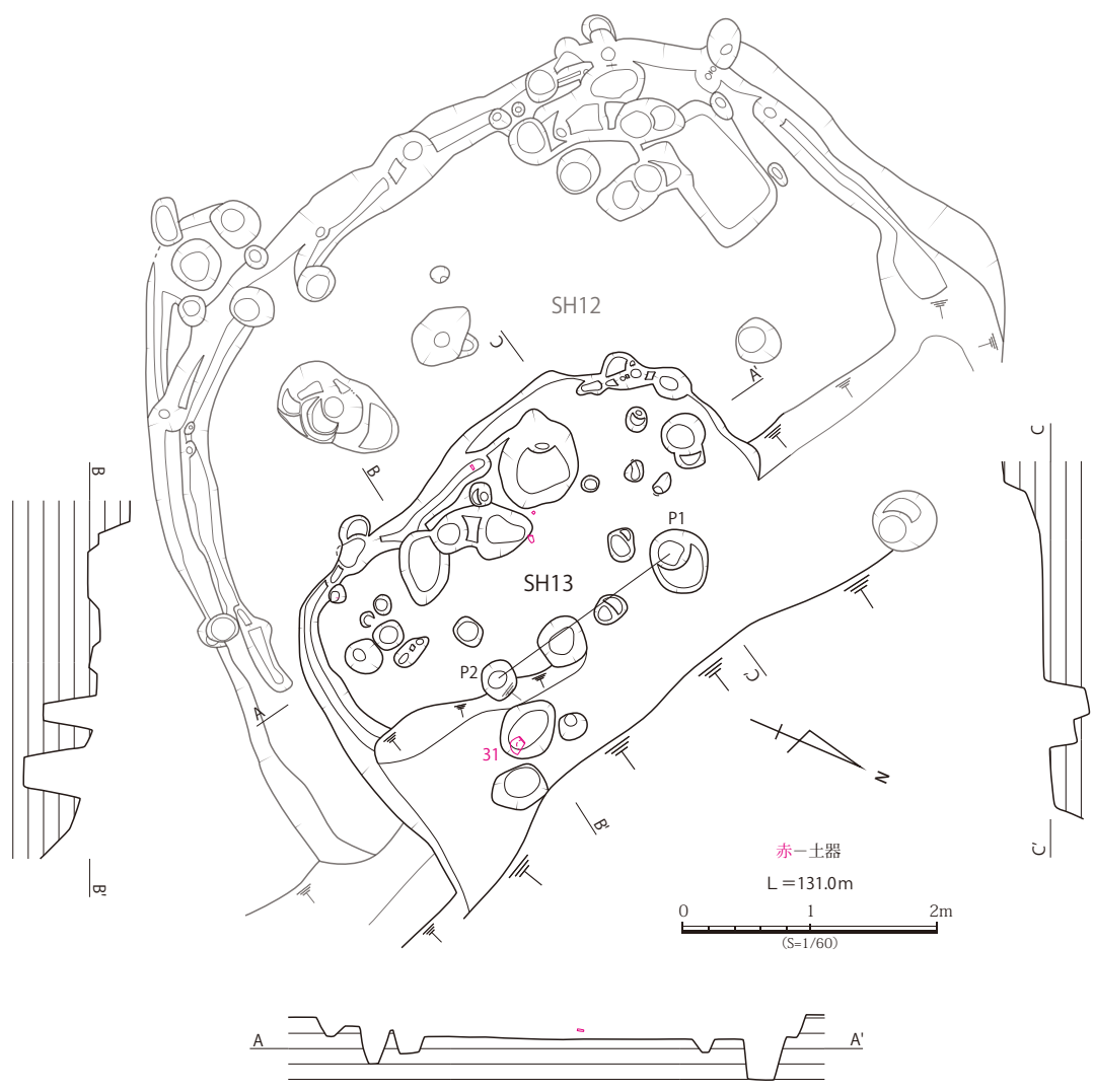
第 135 図 柳遺跡 SH13 実測図 (S=1/60)
