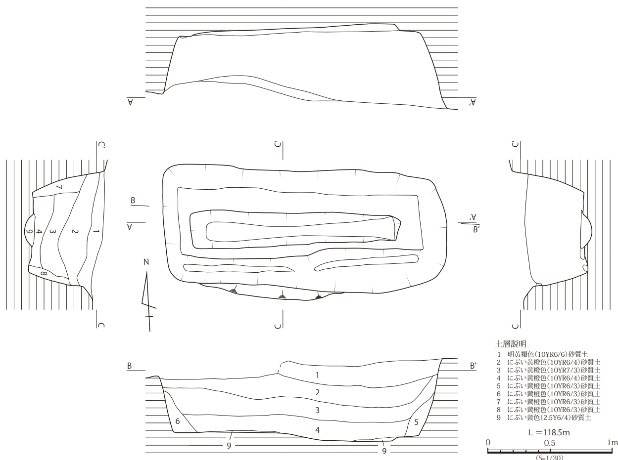
第 101 図 坊主山遺跡 ST11 実測図 (S=1/30)
