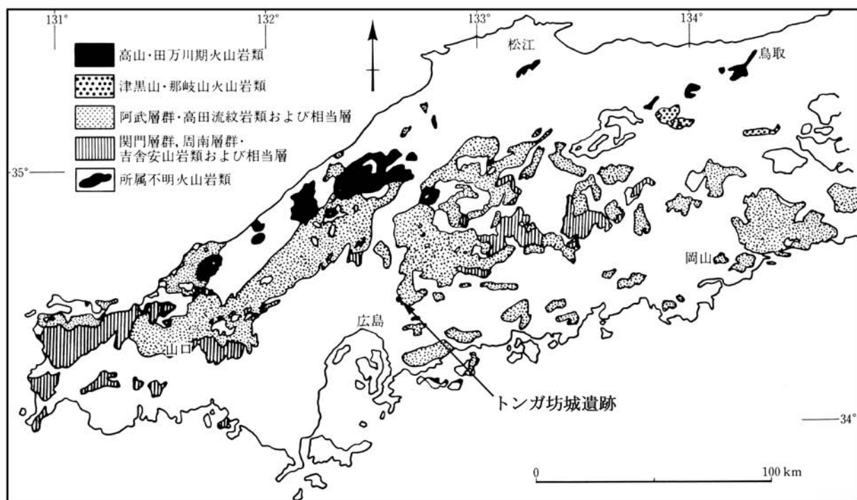
図2 中国地方における白亜紀～古第三紀の火山岩類の分布 (日本の地質『中国地方』編集委員会編, 1991より引用)
