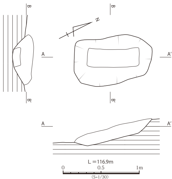
第 97 図 坊主山遺跡 ST6 実測図
