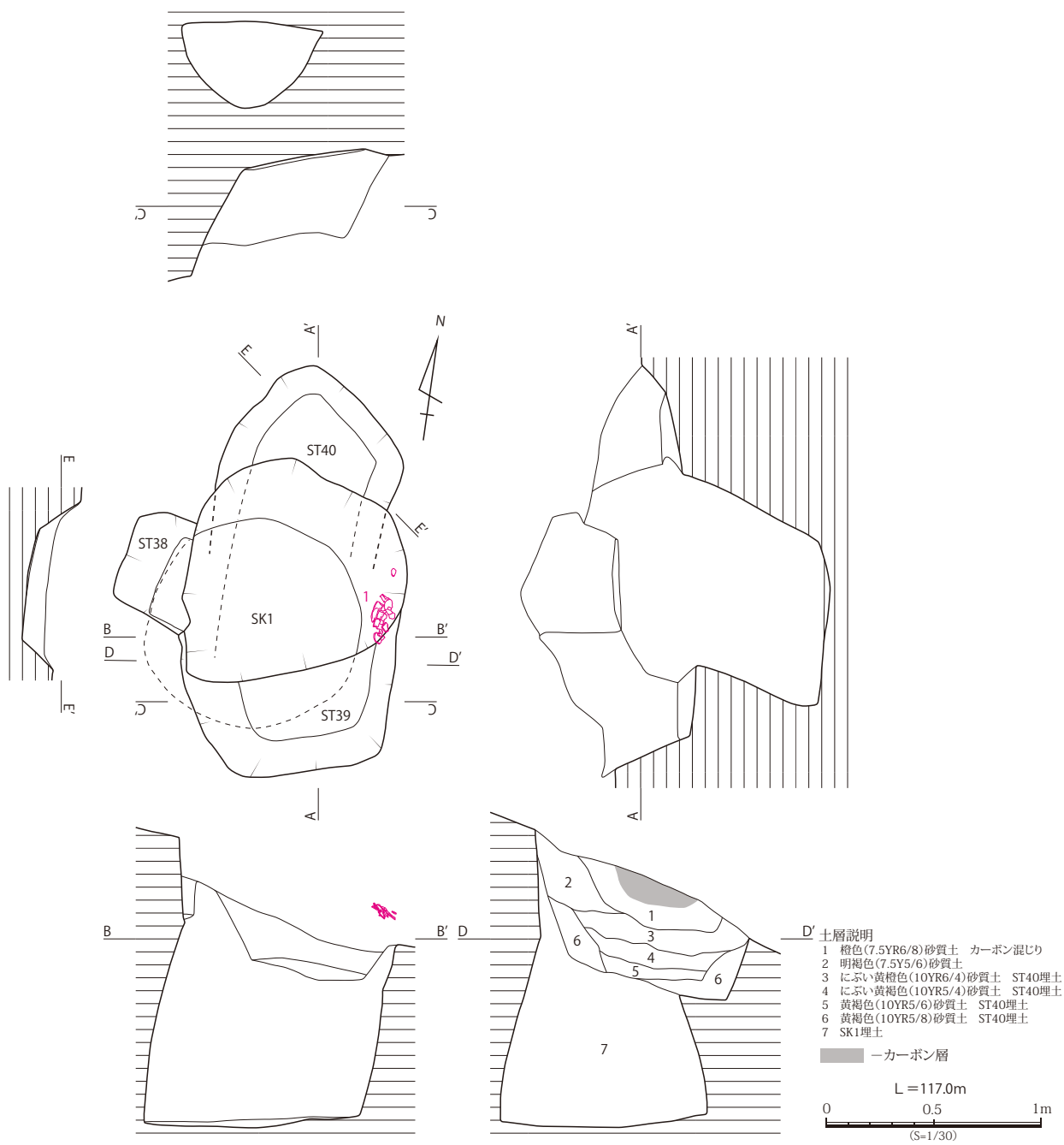
第 121 図 坊主山遺跡 ST39・ST40・SK1 実測図 (S=1/30)
