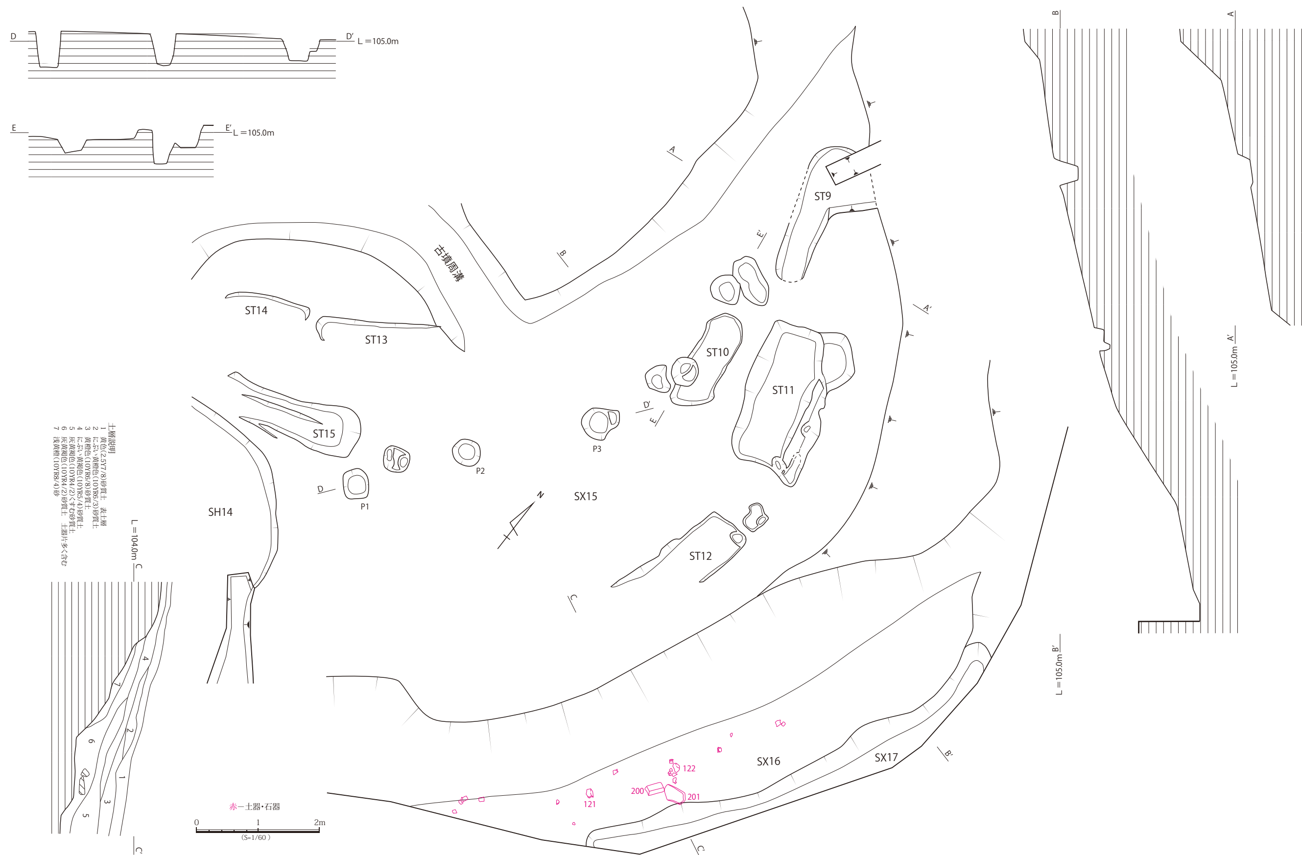
第 45 図 トンガ坊城遺跡 SX15・SX16・SX17 実測図 (S=1/60)
