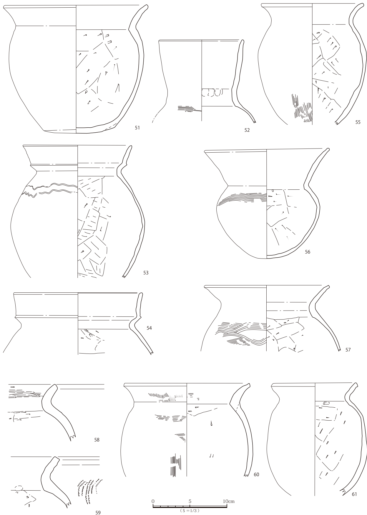
第 65 図 出土遺物実測図 (6) (S=1/3)
