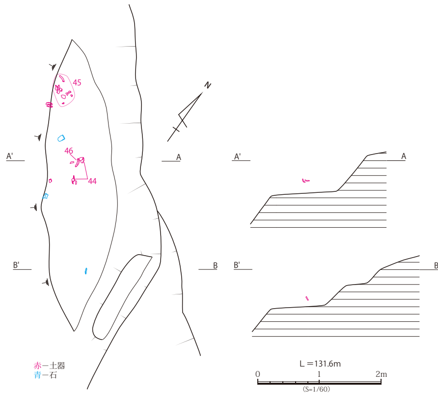
第 137 図 柳遺跡 SX2 実測図 (S=1/60)
