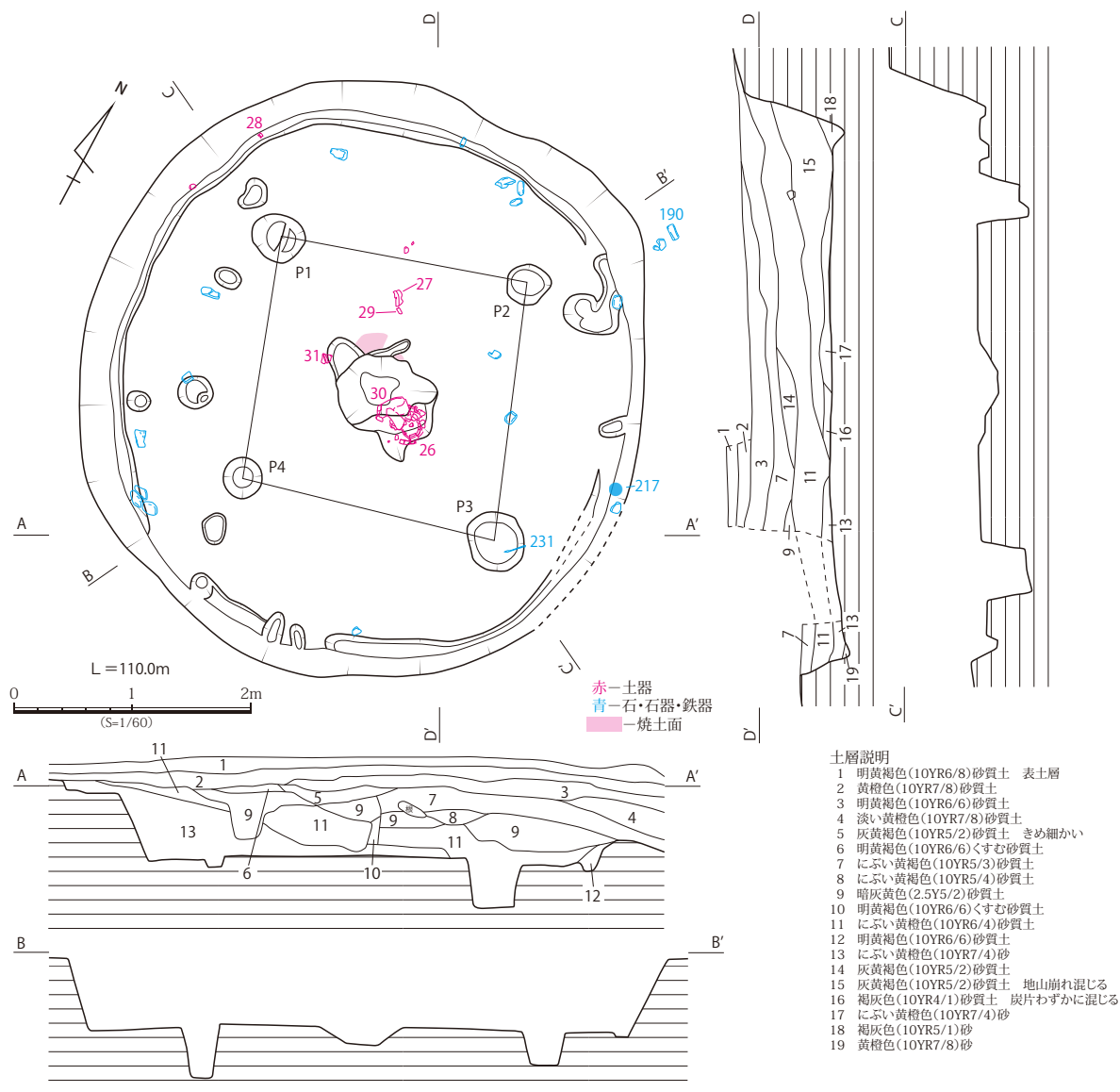
第 29 図 トンガ坊城遺跡 SH12 実測図 (S=1/60)
