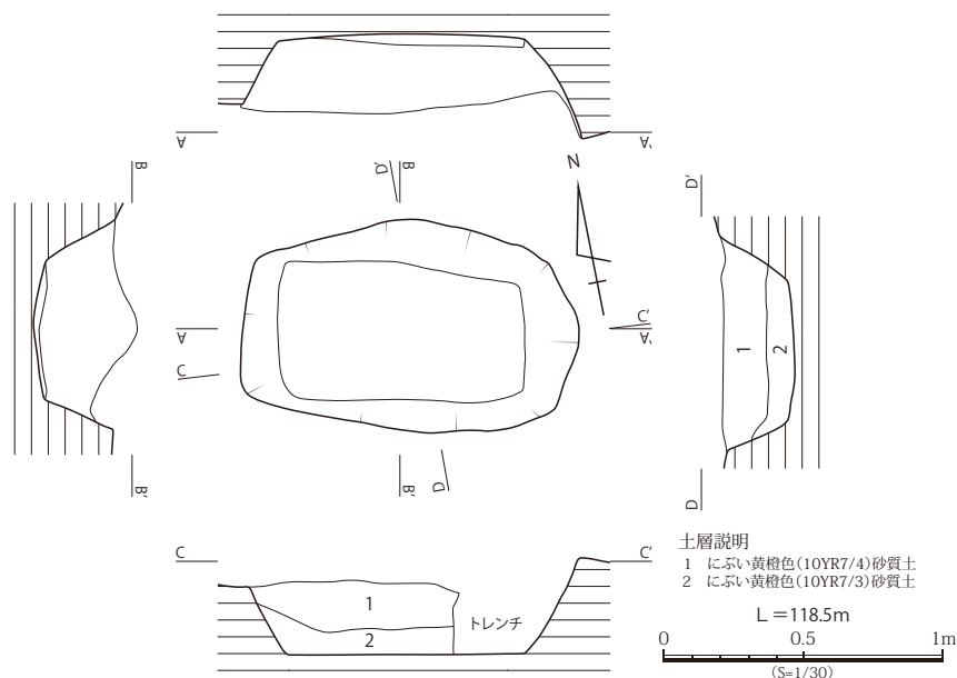
第 99 図 坊主山遺跡 ST8 実測図 (S=1/30)
