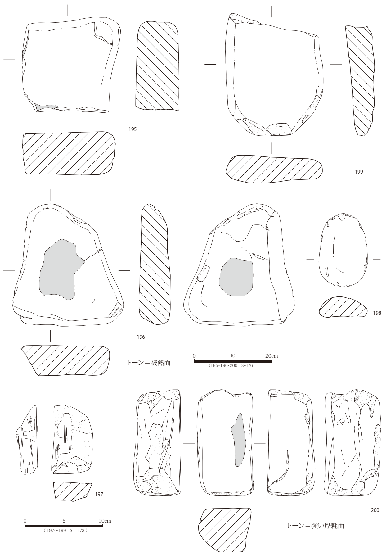
第 76 図 出土遺物実測図 (17) (195・196・200 は S=1/6, 他は S=1/3)
