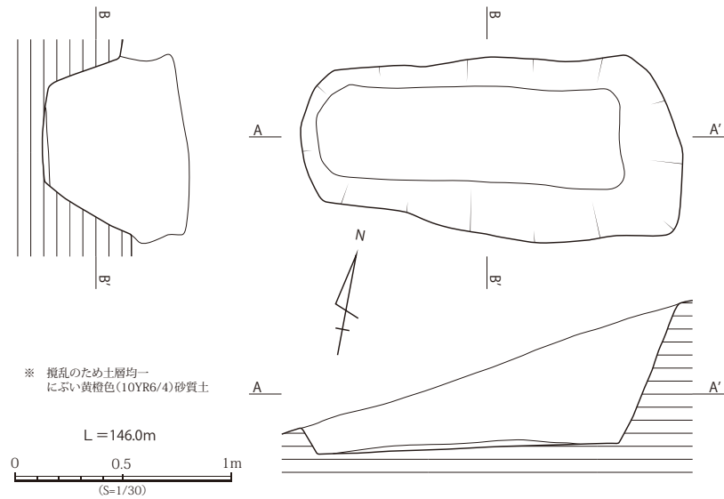
第 178 図 琴平遺跡 ST15 実測図 (S = 1/30)
