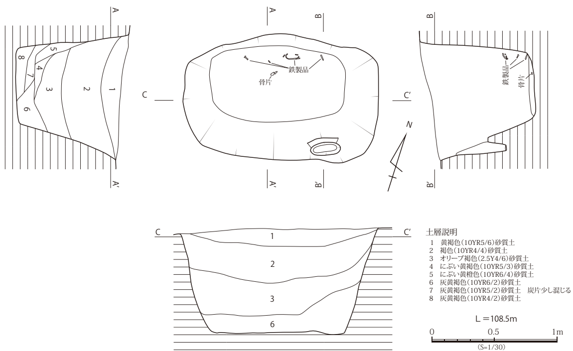
第 89 図 ST22 実測図 (S=1/30)
