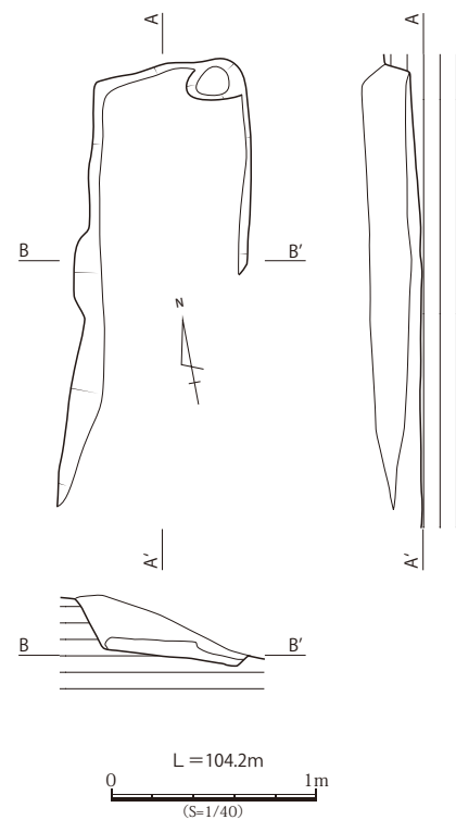
第 57 図 ST12 実測図 (S=1/40)
