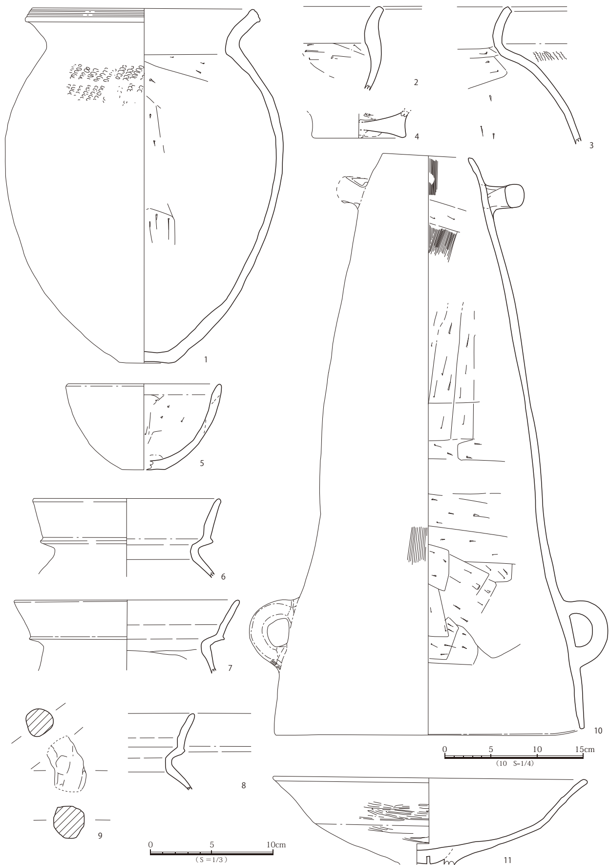
第 60 図 出土遺物実測図 (1) (S=1/3, 10 は S=1/4)
