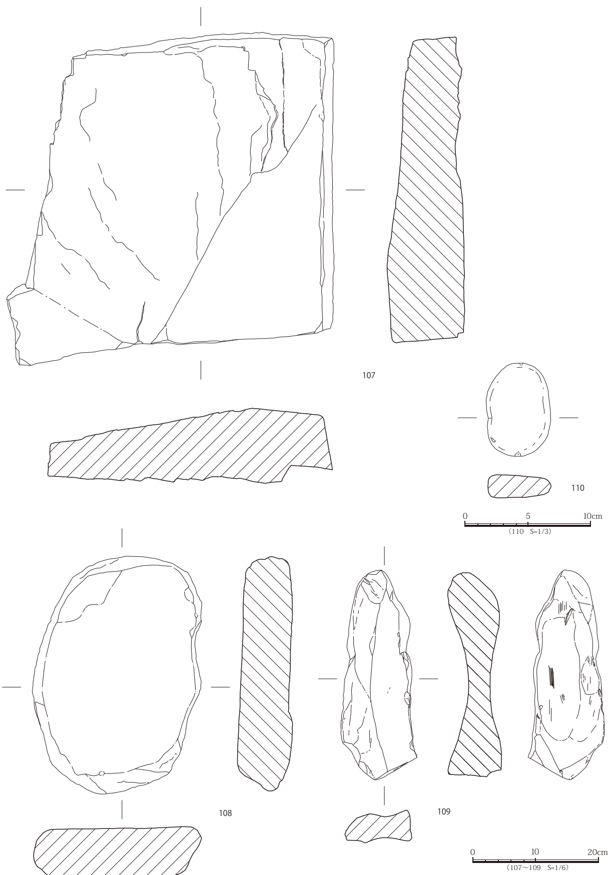
第 159 図 出土遺物実測図 (11) (107 ~ 109 は S=1/6, 110 は S=1/3)
