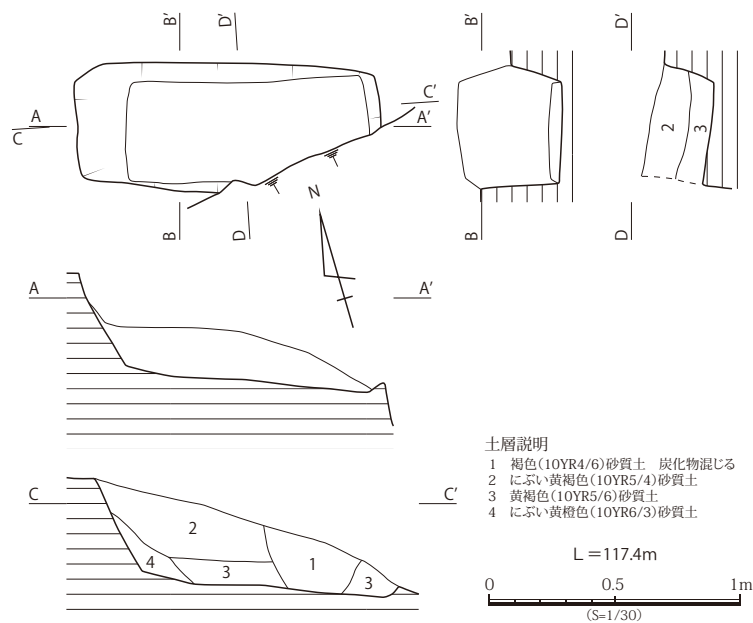
第 120 図 坊主山遺跡 ST38 実測図 (S=1/30)
