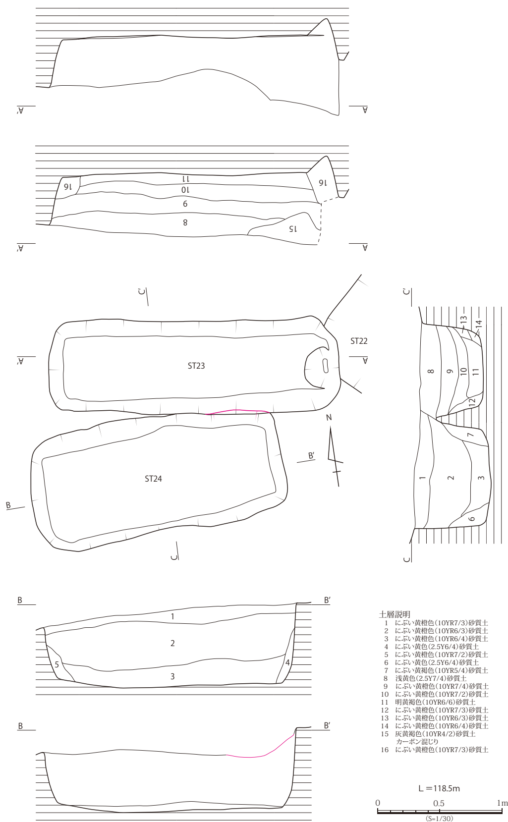
第 111 図 坊主山遺跡 ST23・ST24 実測図 (S=1/30)
