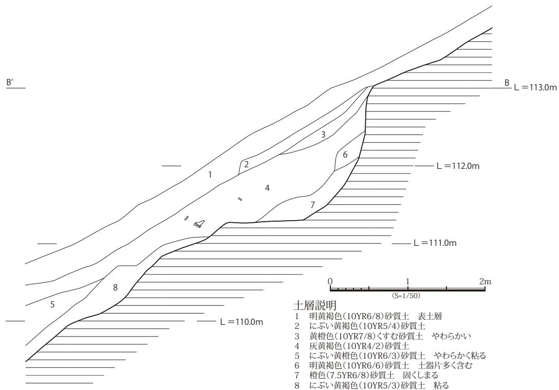
第 86 図 トンガ坊城跡豎堀状遺構 B－B′ 土層断面図 (S=1/50)
