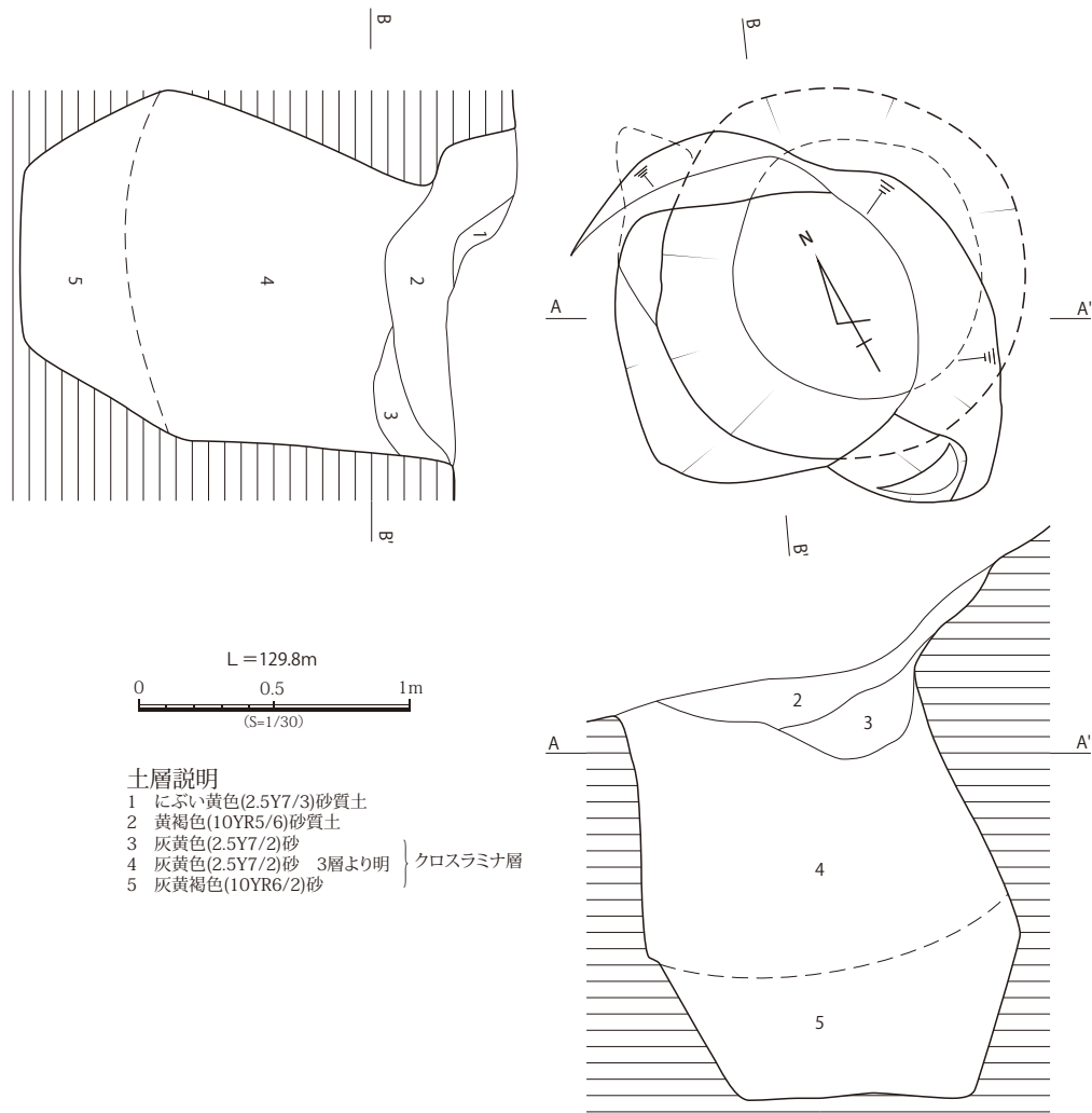
第 147 図 柳遺跡 SK9 実測図 (S=1/30)
