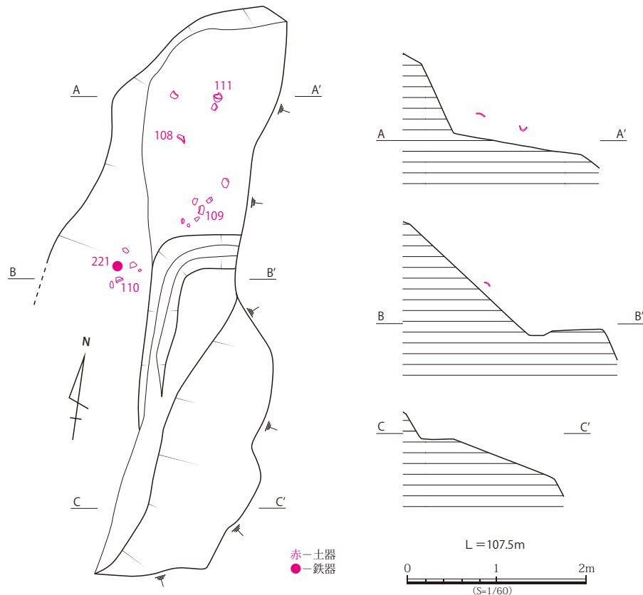
第 37 図 トンガ坊城遺跡 SX12 実測図 (S=1/60)
