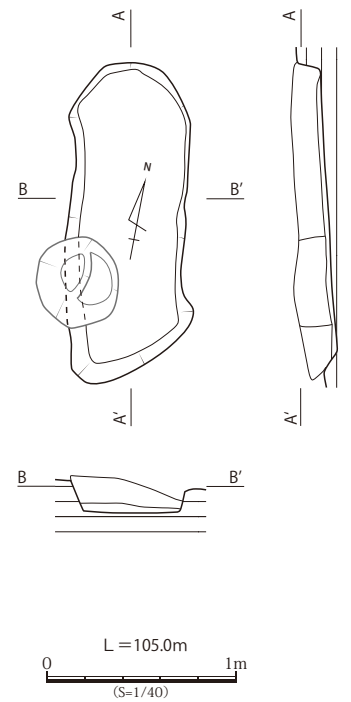
第 55 図 ST10 実測図 (S=1/40)
