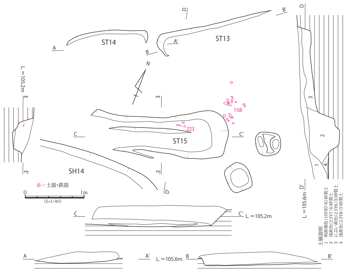
第 58 図 ST13・ST14・ST15 実測図 (S=1/40)
