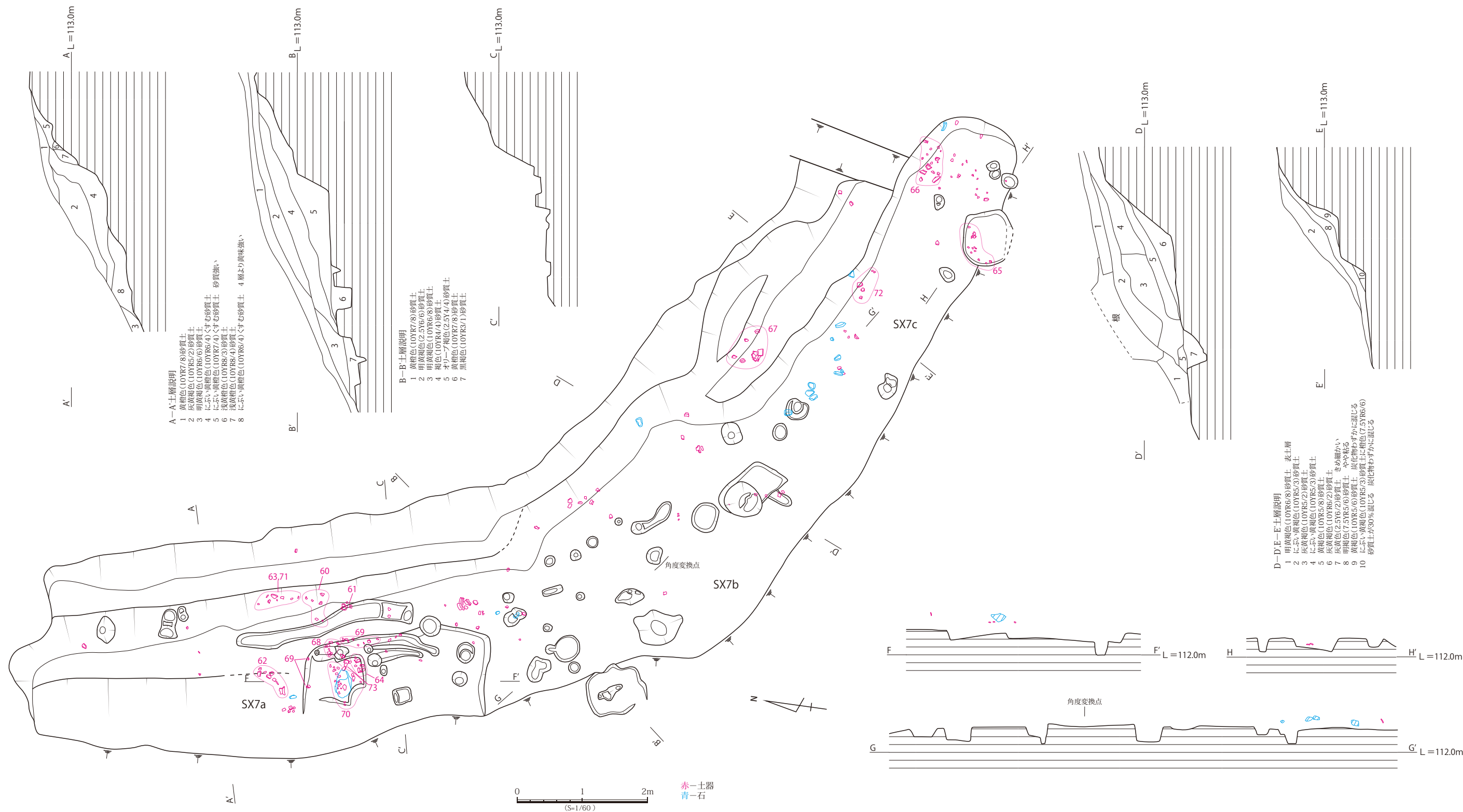
第 28 図 トンガ坊城遺跡 SX7 実測図 (S=1/60)
