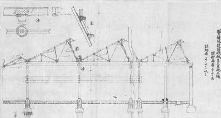
製缶場通調機械室及其他工場縦断面図 青図を反転 当館蔵
