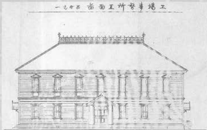
工場事務所正面図 青図を反転 当館蔵
