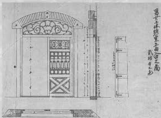
男女工休館室正面入口之図 青図を反転 当館蔵
