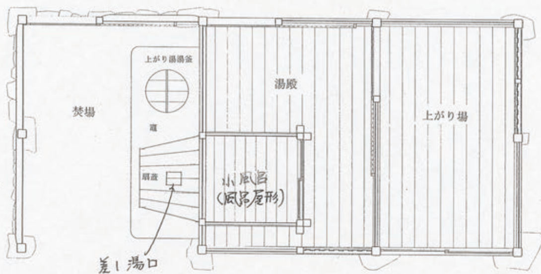
広島県山県郡千代田町 万徳院風呂屋・屋形 平面図
