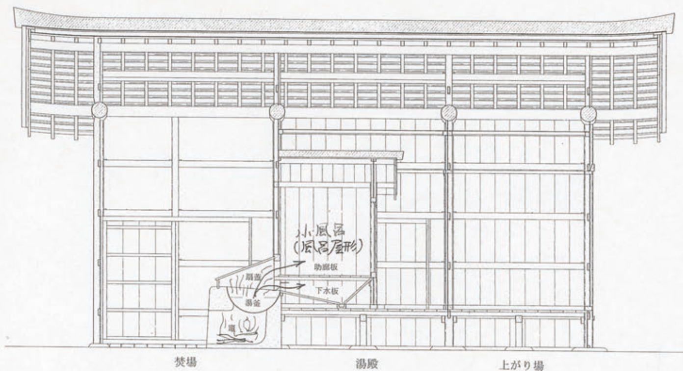
広島県山県郡千代田町 万徳院風呂屋・屋形 桁行断面図
