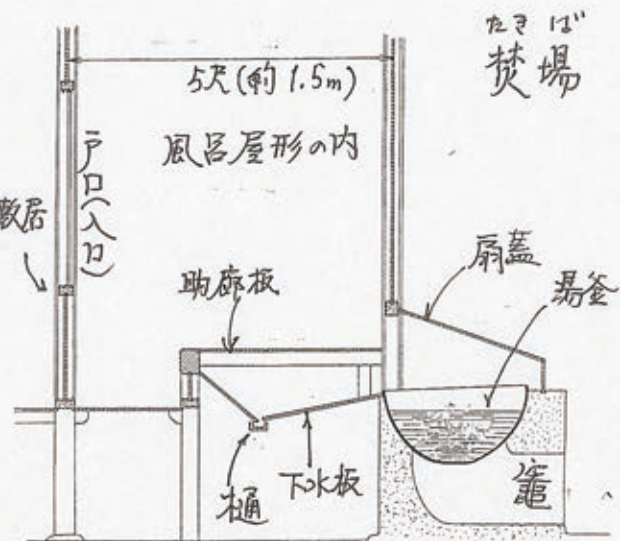
風呂の構造(『愚子見記』から作成)
