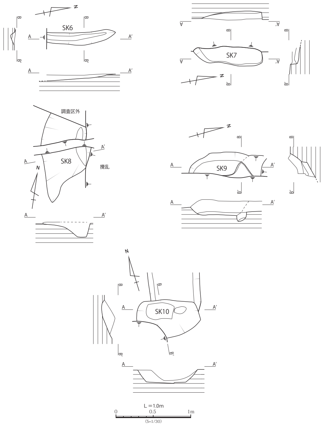
第 5 図 SK6・SK7・SK8・SK9・SK10 実測図 (S=1/30)
